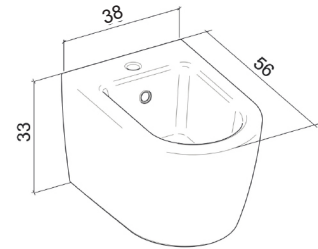
DIMENSIONI /DIMENSIONS
