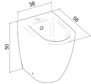
DIMENSIONI /DIMENSIONS
